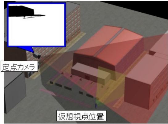
図5：定点カメラ画像上への逆投影結果
